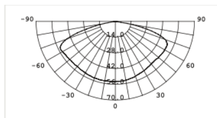
140° Abstrahlwinkel
