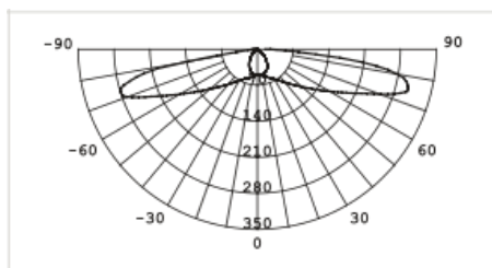
135x55° Abstrahlwinkel
