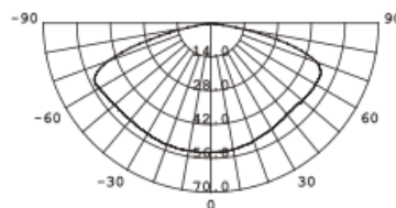
140° Abstrahlwinkel
