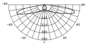
150x70° Abstrahlwinkel
